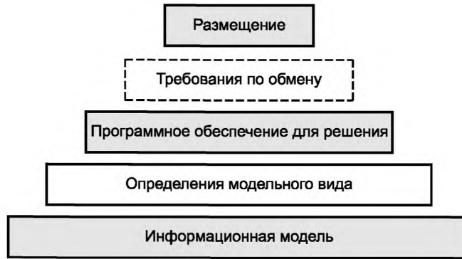
Рисунок А.5 — Слои структуры обмена информацией
