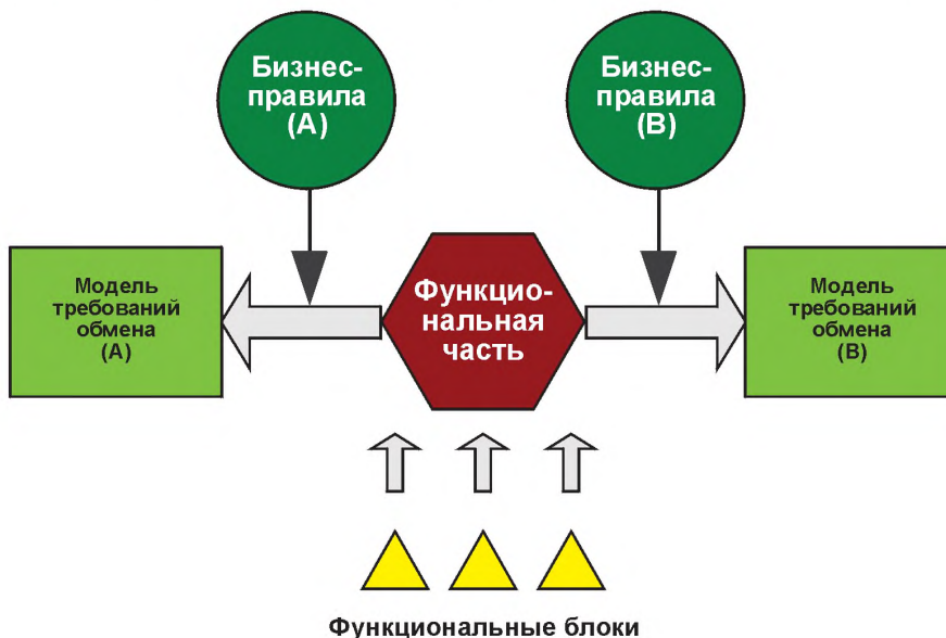
Рисунок 7 — Применение бизнес-правил
