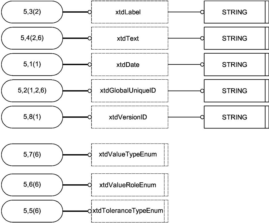
Рисунок 5 — EXPRESS-G диаграмма 5 — Основные типы
