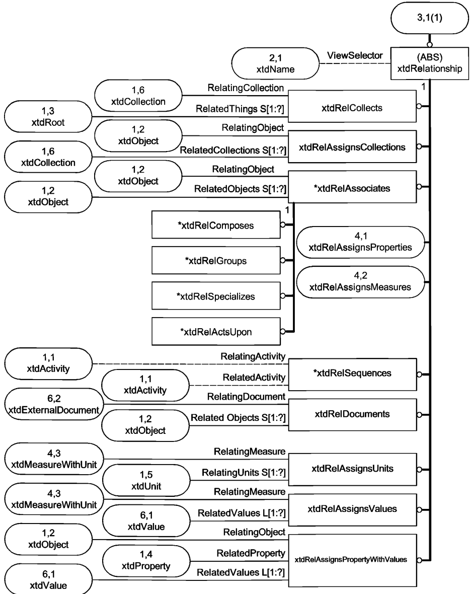
Рисунок 3 — EXPRESS-G диаграмма 3 — Отношения
